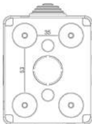
Vista posteriore
