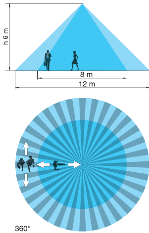
Montaggio su soffitti alti fino a 6 metri
