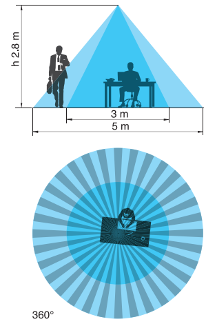
Rilevatore di movimento e di presenza
