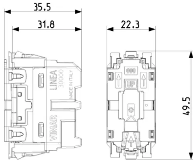
Vista ingombri
