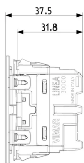
Vista ingombri
