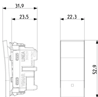
Vista ingombri
