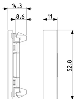
Vista ingombri
