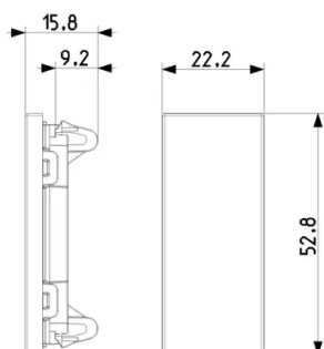
Vista ingombri
